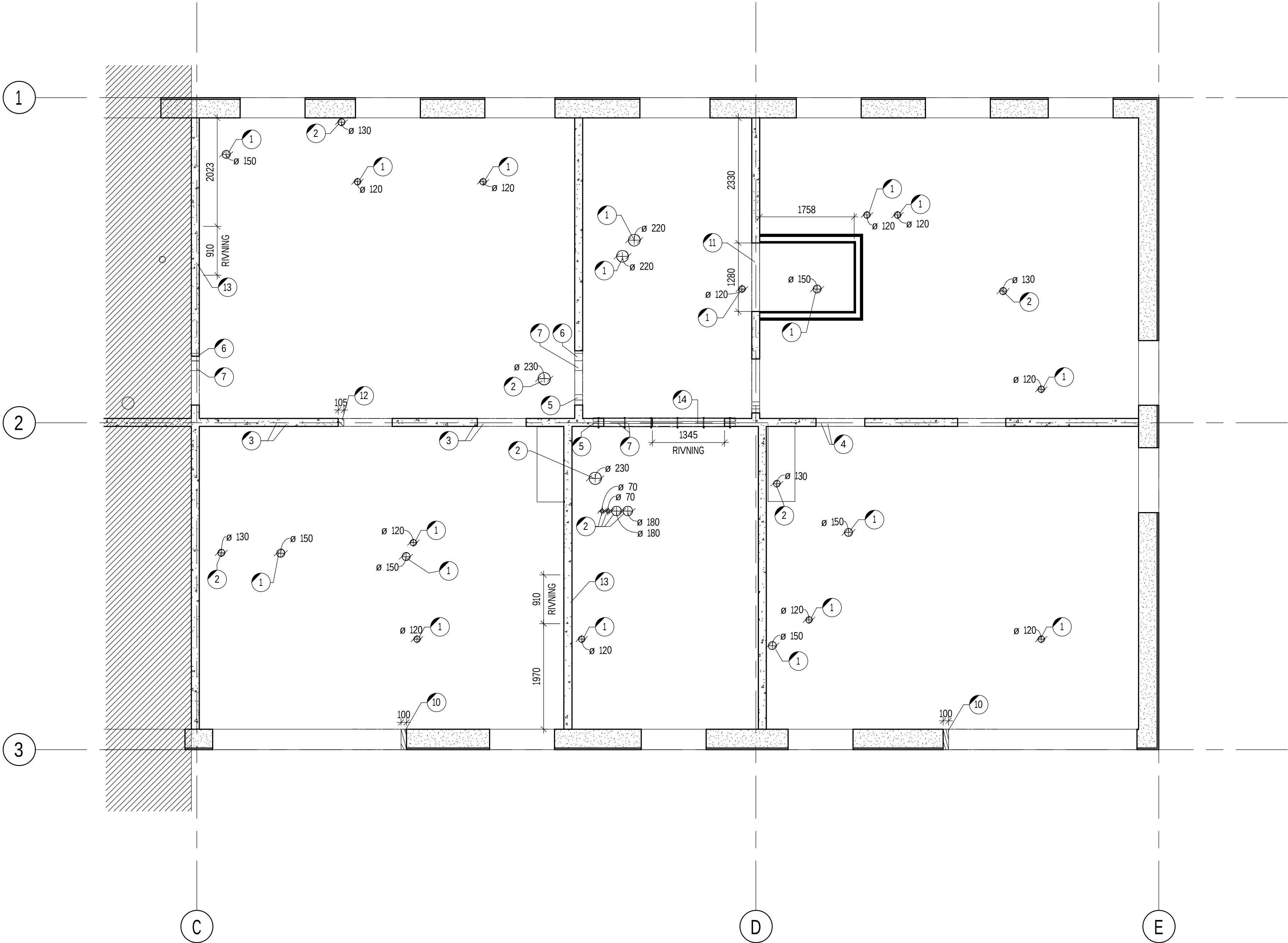
PLAN 2 LÄGENH. - Del 2 1 : 50
